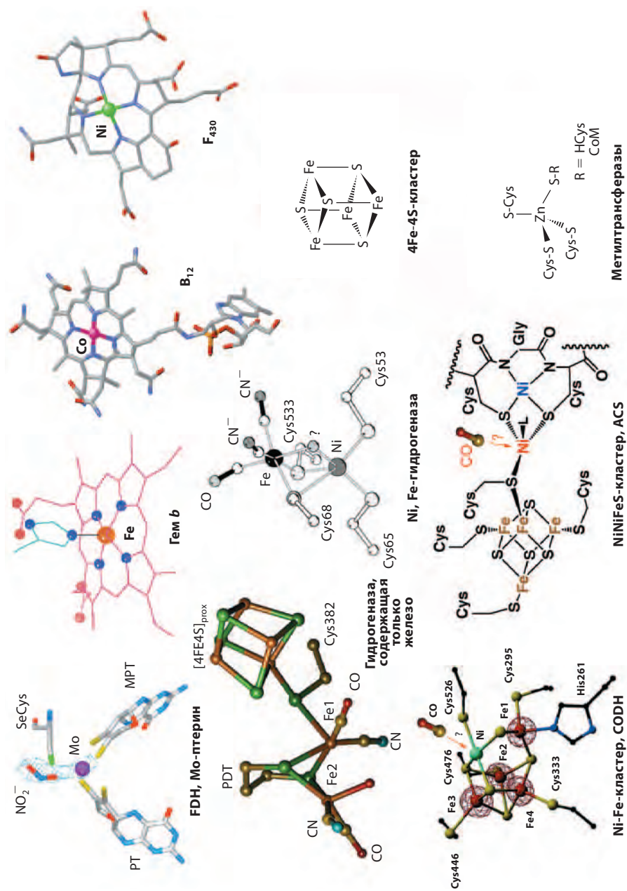
Рис. XII.2.2. Металлсодержащие сайты в путях восстановления одноуглеродных соединений
