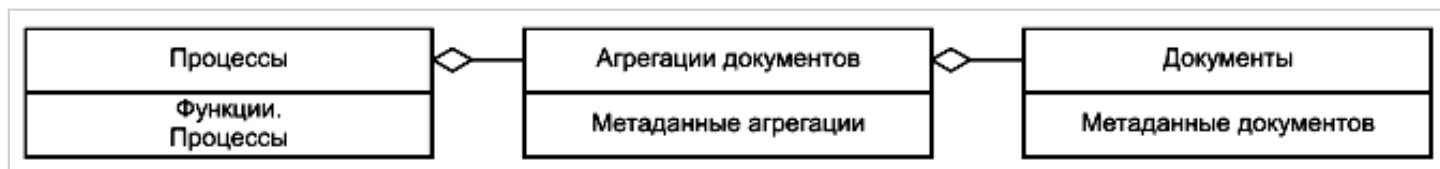
Рисунок 3 - Схема отношений для агрегации "Дело, ед.хр."
