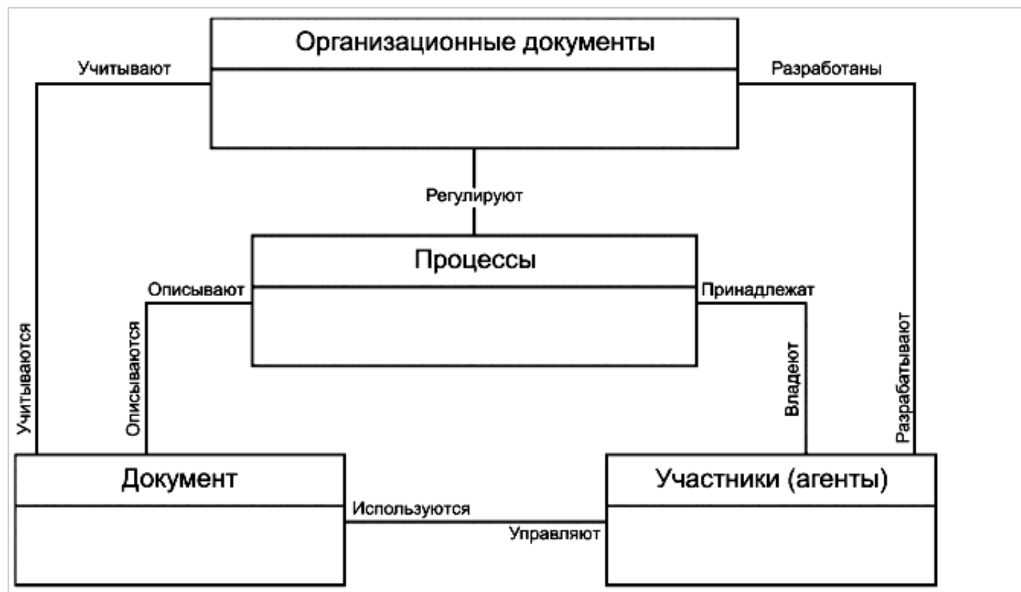
Рисунок 1 - Схема взаимосвязей между объектами (сущностями) метаданных
